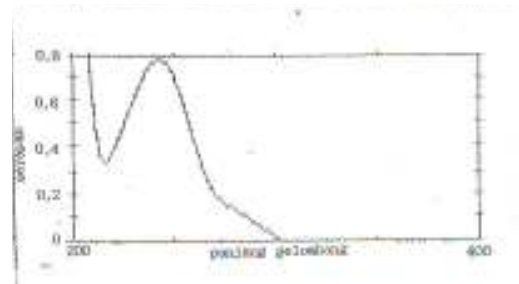
Gambar 4. Spektrum UV larutan bahan baku parasetamol BPF dalam campuran HCL 0,1 N dalam metanol ( 1 dalam 100)
