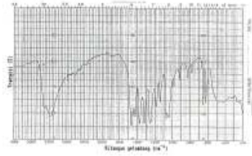
Gambar 2. Spektrum infra merah bahan baku pembeding Parasetamol BPF
