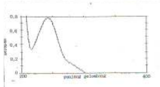
Gambar 3. Spektrum UV larutan bahan baku parasetamol dalam campuran HCl 0,1 N dalam metanol (1 dalam 100).
