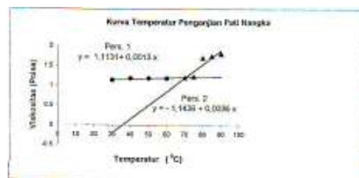
Gambar 8. Kurva temperatur penganjian pati nangka
